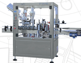
OMB / Z-Italia Etikettierer 1.000 Fl/h bis 50.000 Fl/h
