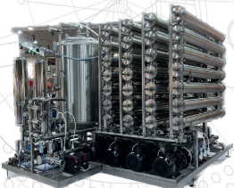
Osmose u. Entalkoholisierung kombinierte Modulbauweise
