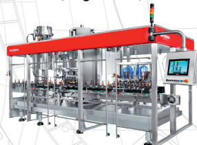
Bertolaso Füller 1.500 Fl/h bis 50.000 Fl/h
